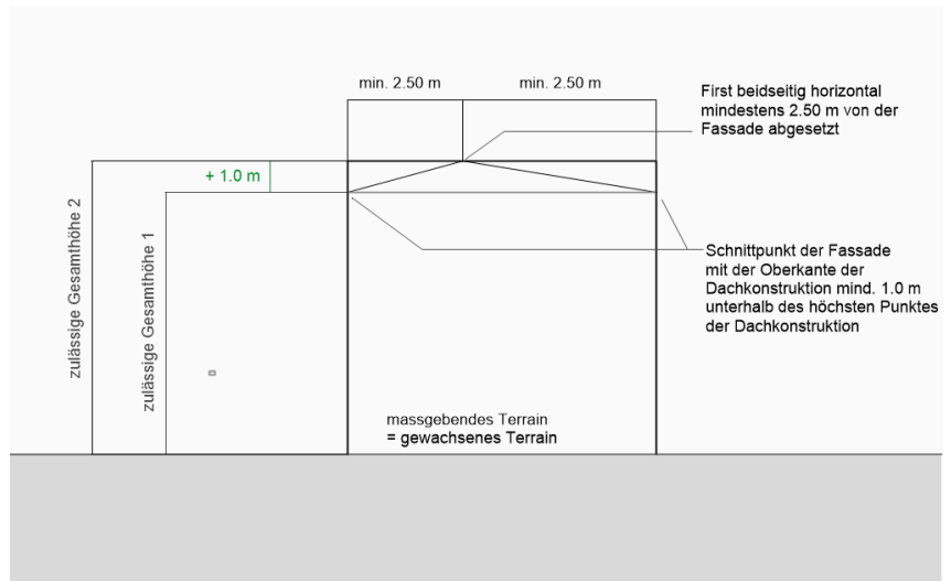
Abbildung 10: zulässige Gesamthöhe mit Schrägdachbonus
